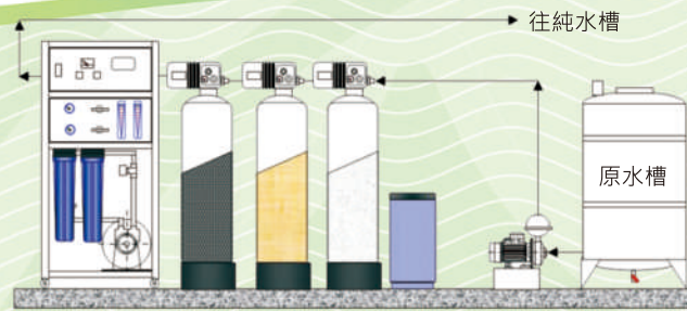
系統標準安裝圖示
